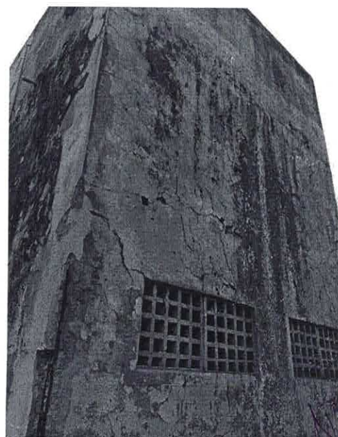
Revestimentos externos com graves infiltrações, causando desprendimento.
