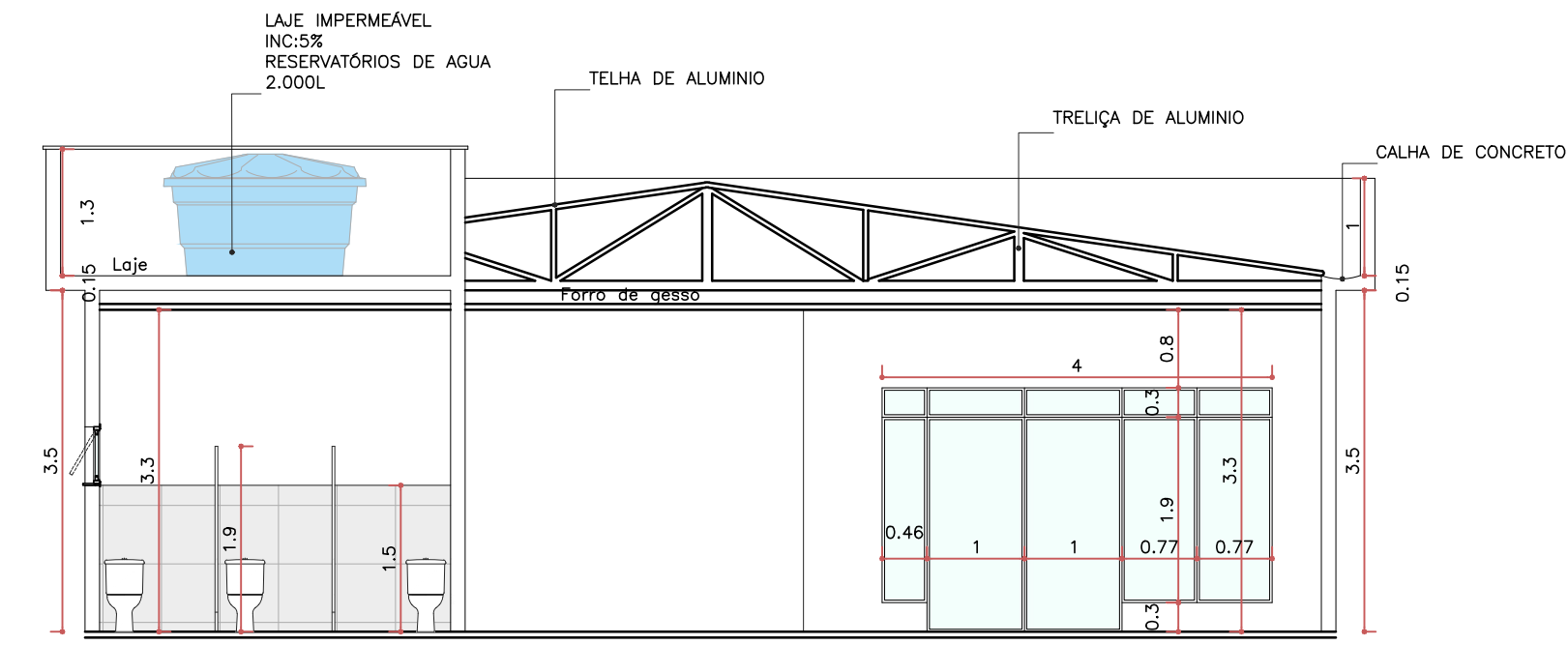
CORTE BB ESC. 1:75
