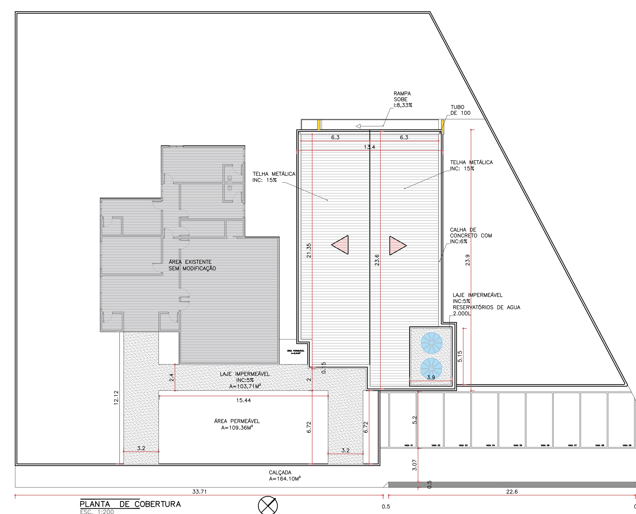
PLANTA DE COBERTURA ESC. 1:200
